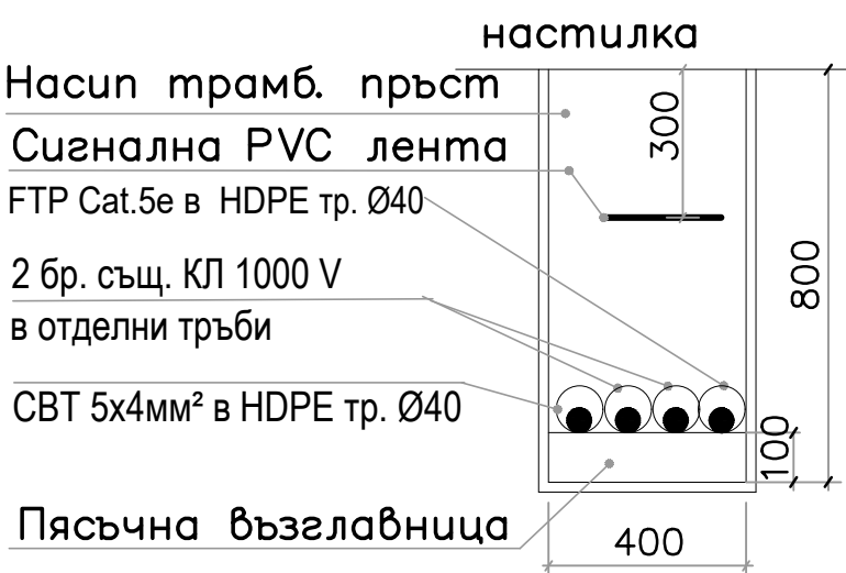
Разрез 1-1
